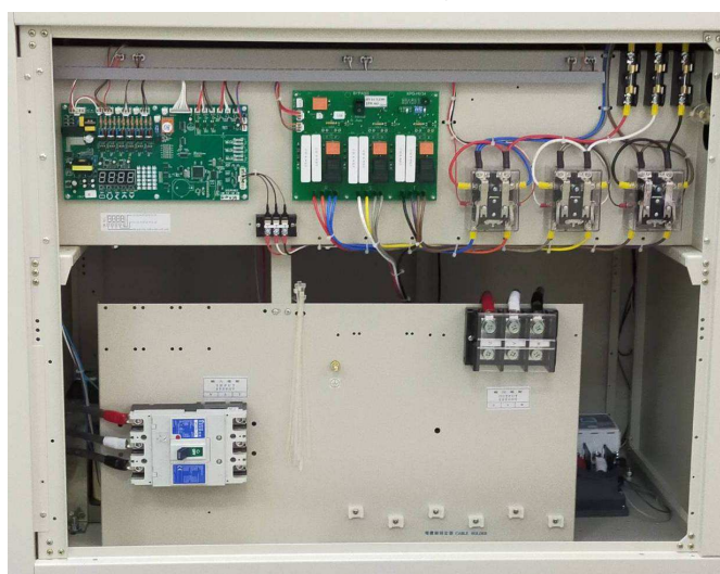
I/P, O/P 接線面
